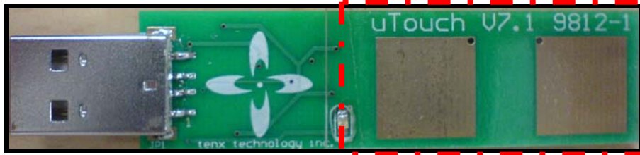
圖 2 兩鍵式觸控感感應區
