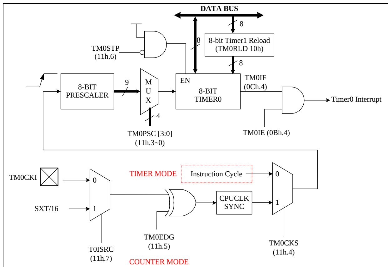
Timer0 框图
