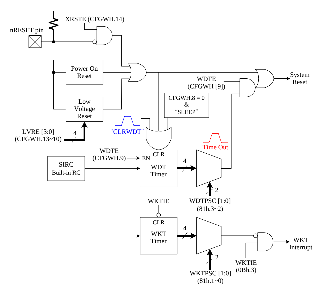
WDT/WKT 框图
