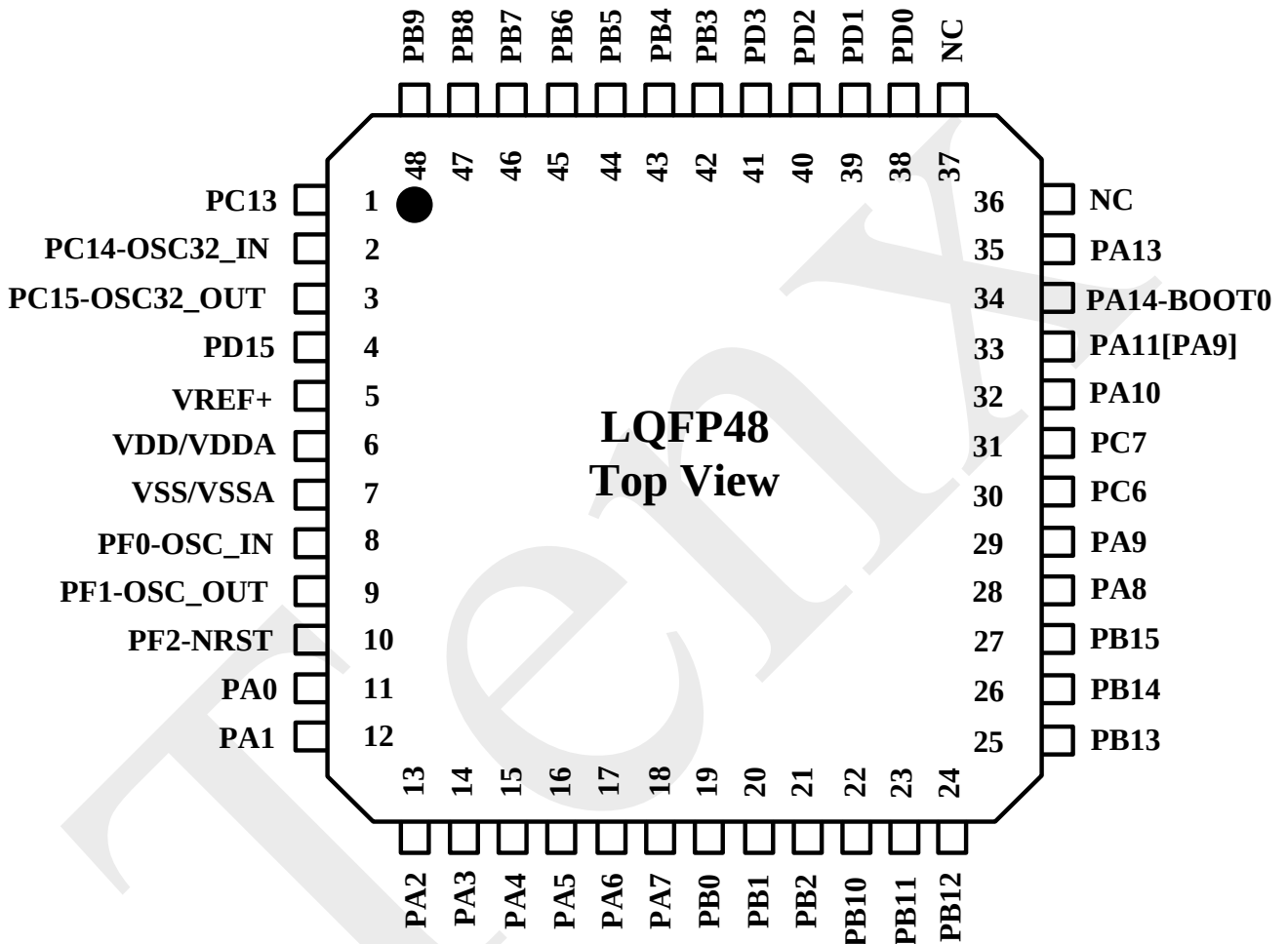
图 4-1-1 TM32M05169LA2 LQFP48 引脚分配图
