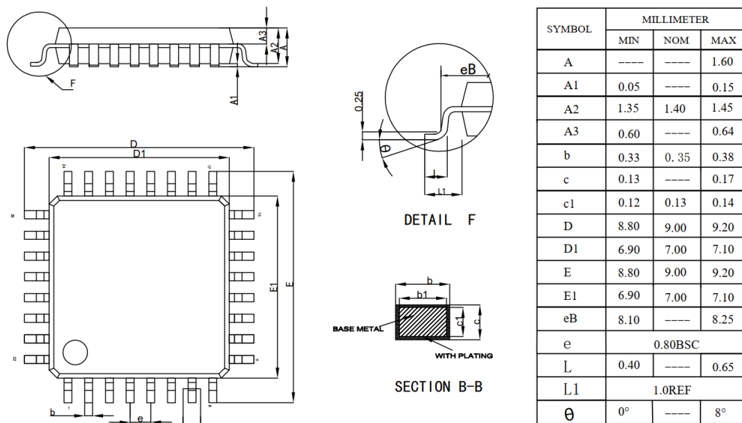
图 6-2 LQFP32-7x7mm 封装外形尺寸数据
