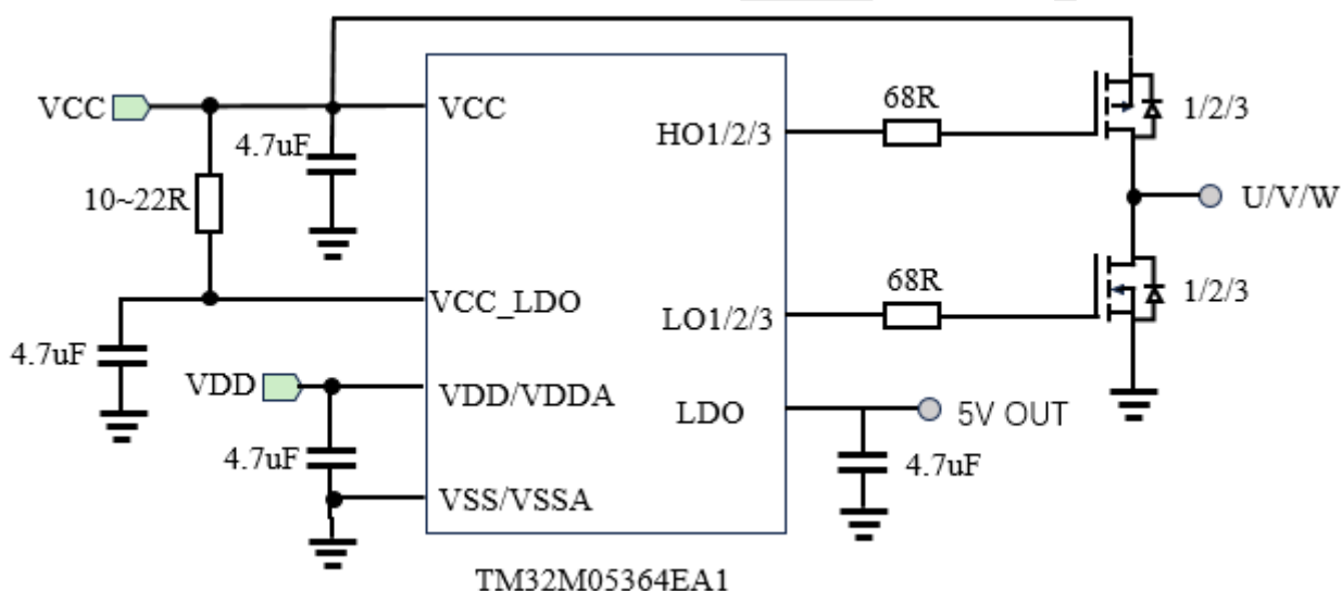
图 5-3-23-1 典型应用电路
