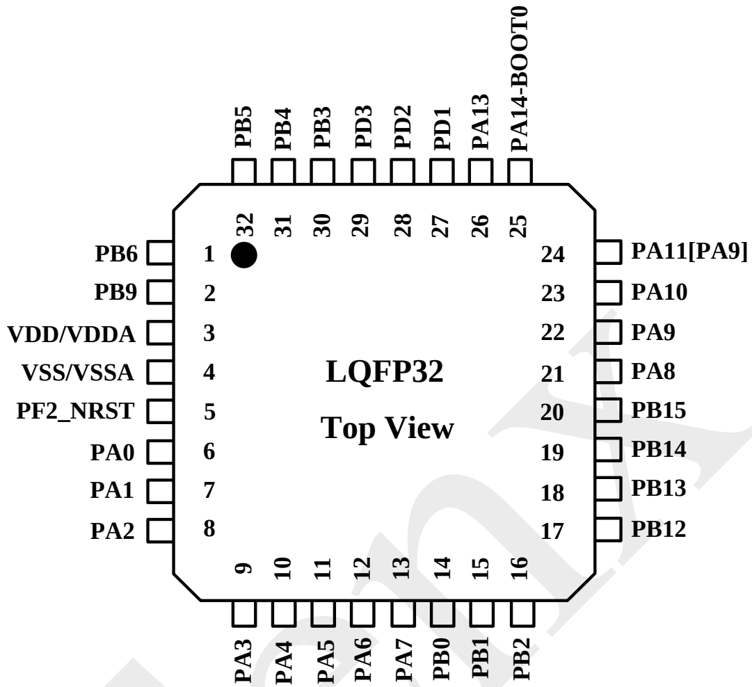
图 4-1-2 TM32M05166LA1 LQFP32 引脚分配图
