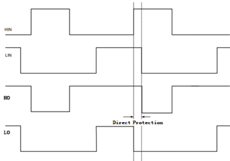
图 5-3-23-2 栅极驱动极性示意图
