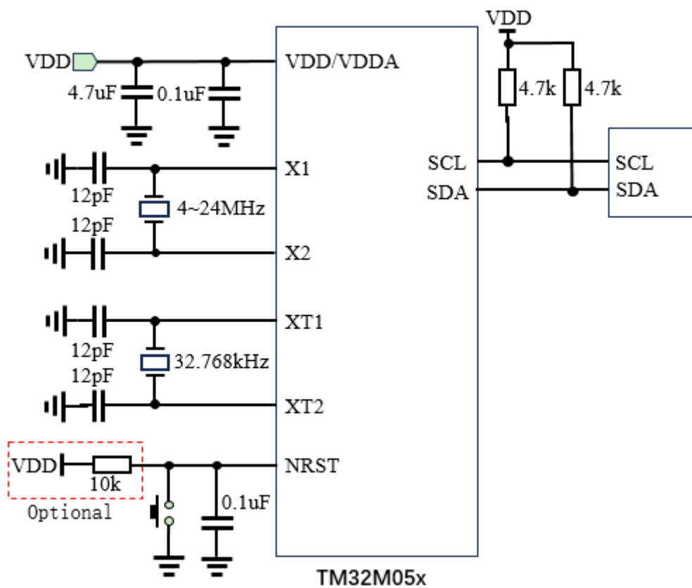
图 5-1-8 TM32M05x 典型应用电路
