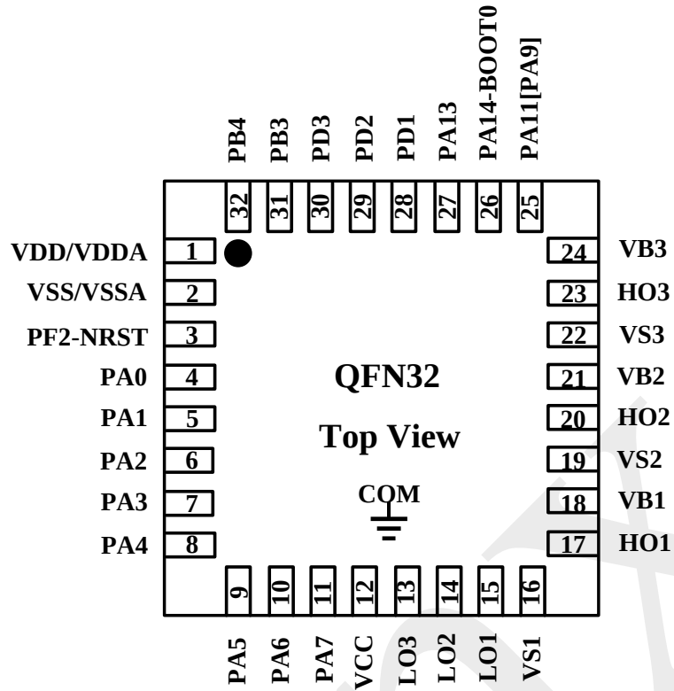
图 4-1-5 TM32M05266UA QFN32 5mm*5mm 引脚分配图
