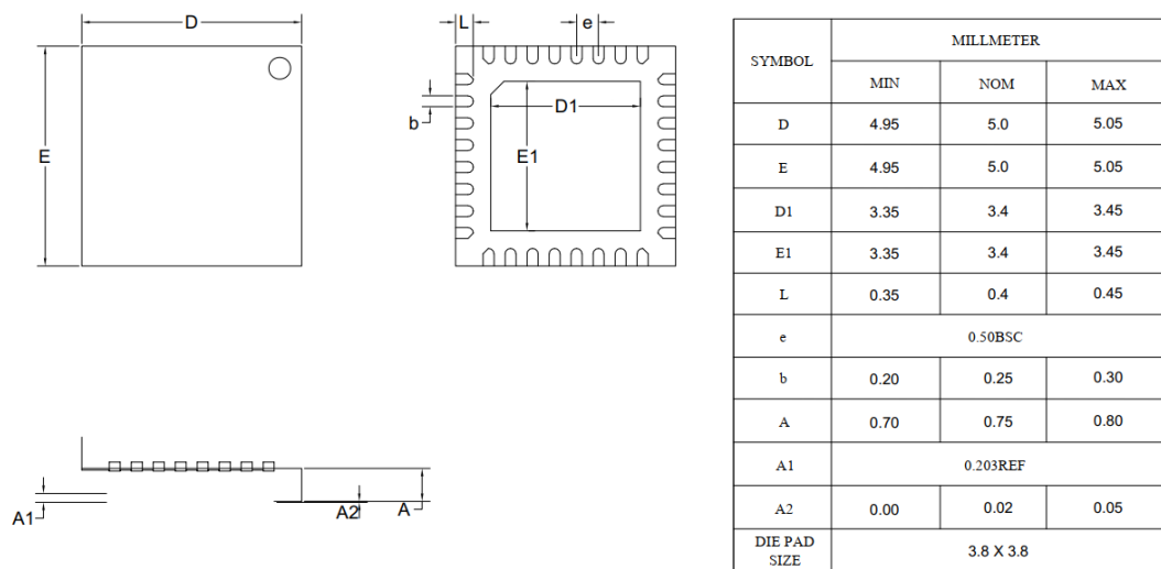
图 6-5 QFN32-5mm*5mm 封装外形尺寸数据
