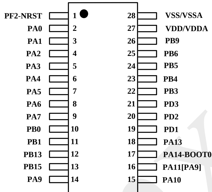
图 4-1-3 TM32M05165TA TSSOP28 引脚分配图
