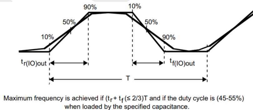
图 5-3-13-1 I/O AC 特性定义
