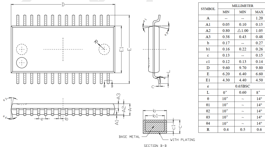
图 6-3 TSSOP28 封装外形尺寸数据
