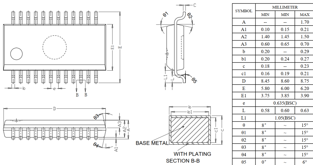
图 6-4 SSOP24 封装外形尺寸数据
