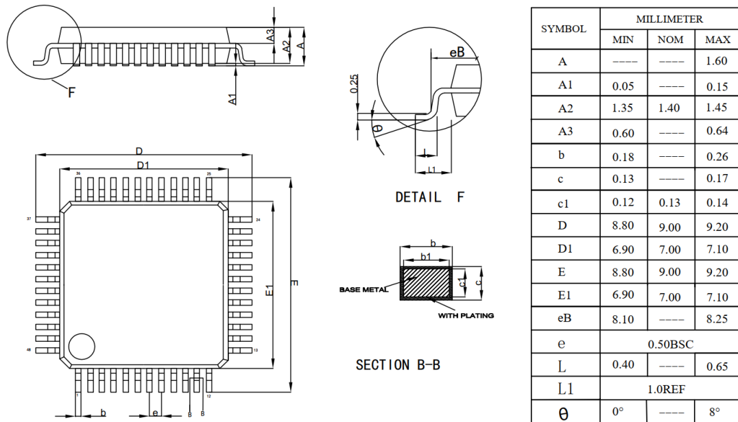
图 6-1 LQFP48-7x7mm 封装外形尺寸数据
