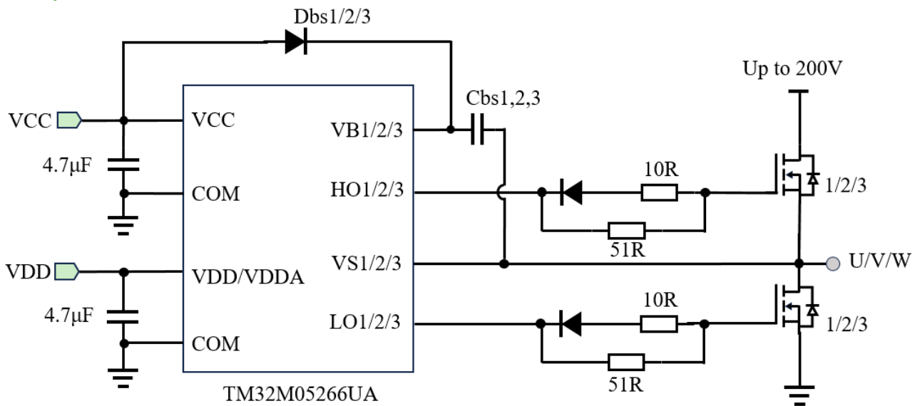
图 5-3-22-1 典型应用电路
