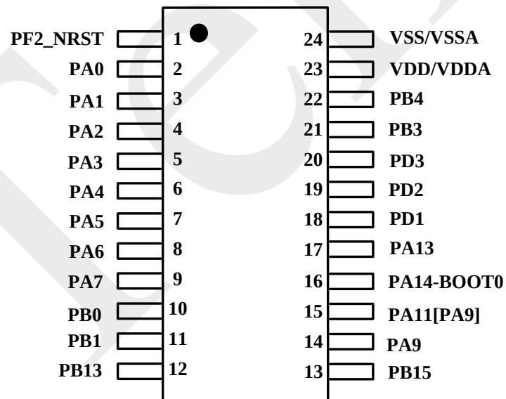
图 4-1-4 TM32M05164EA SSOP24 引脚分配图
